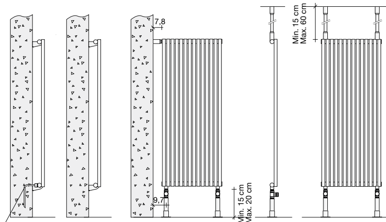
Supporto STANDARD A MURO (cod. ST)
