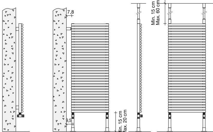
Supporto STANDARD A MURO (cod. ST)
