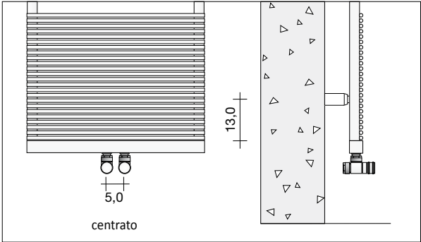
Schema tecnico allacciamento BA10 i5
