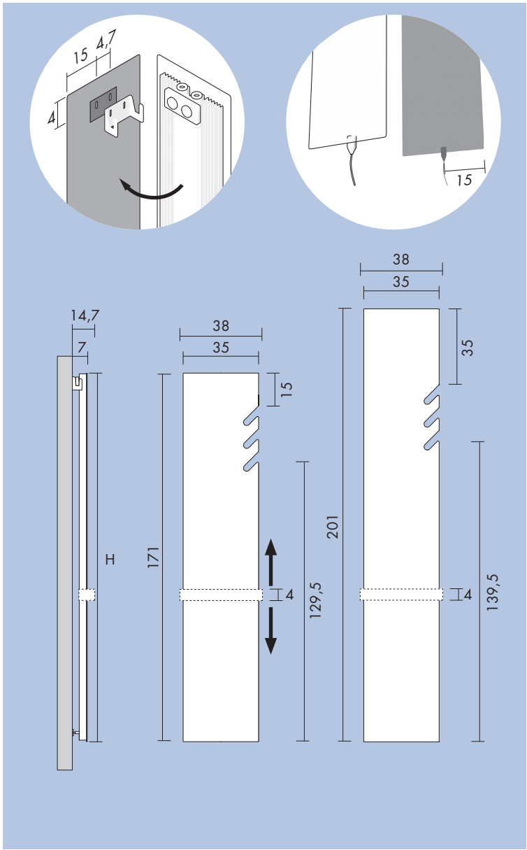
Electric with schuko plug / Version électrique avec prise schuko / Elektromodell mit schukosteckdose / Versión electrica con enchufe schuko
