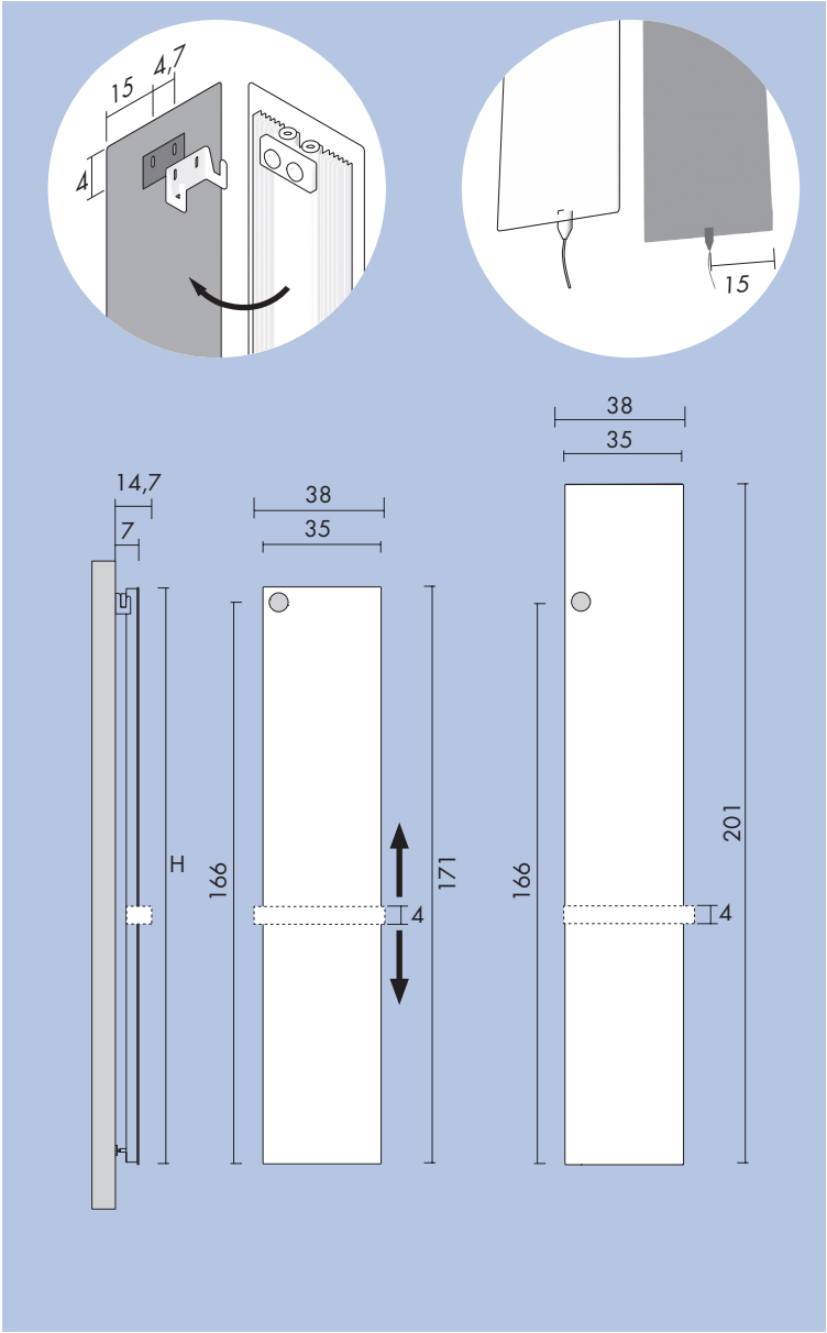
Electric with schuko plug / Version électrique avec prise schuko / Elektromodell mit schukosteckdose / Versión eléctrica con enchufe schuko
