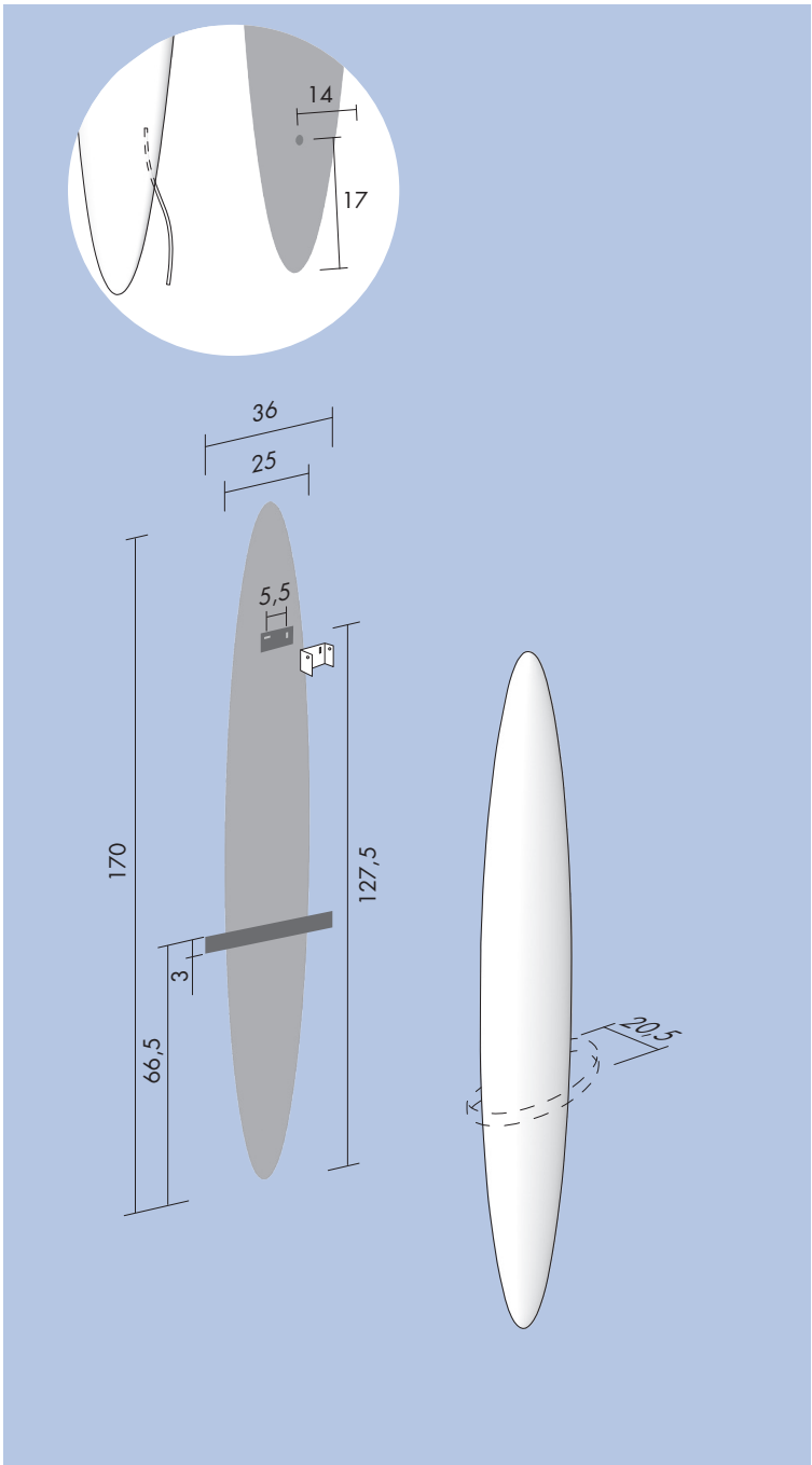
Electric with cable / Version électrique avec cable / Elektrische Ausführung mit Kabel / Versión electrica con cable
